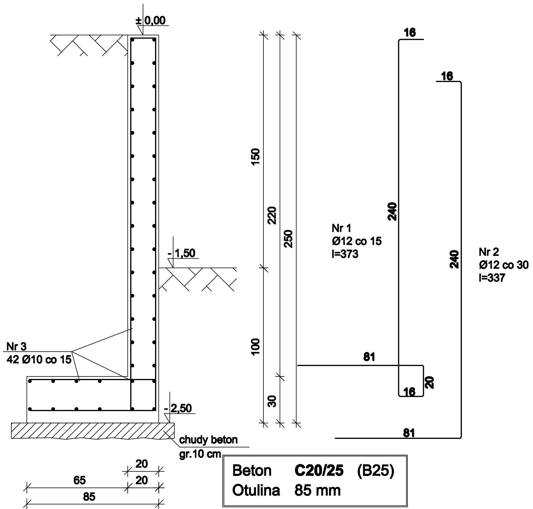
Wykaz zbrojenia dla ściany dł. 42,10m
