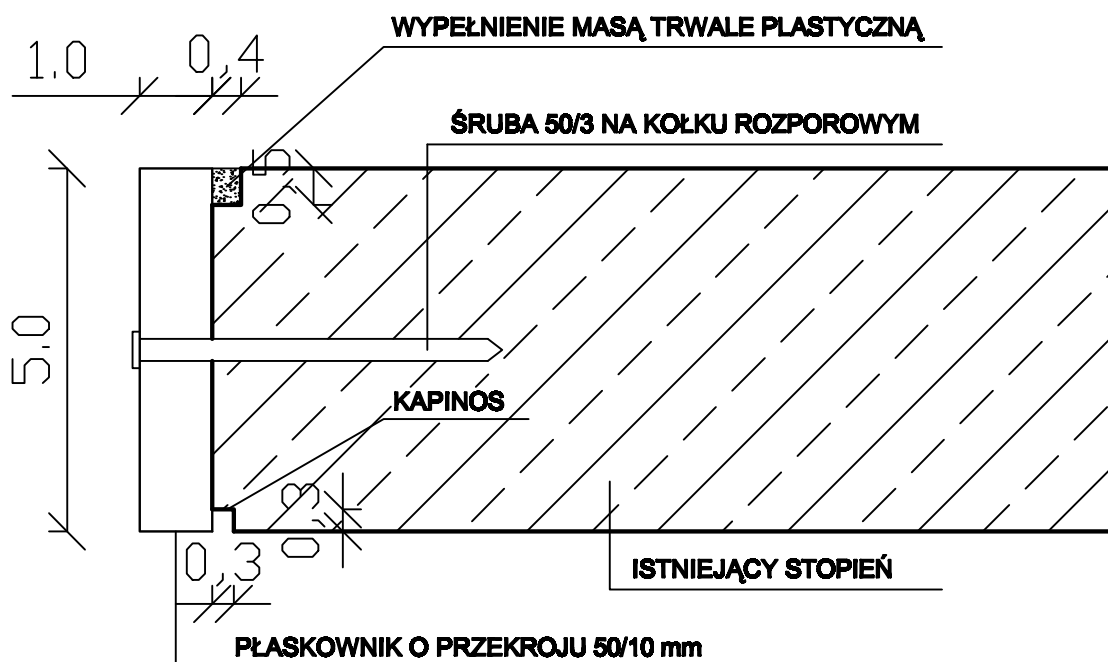
PRZEKRÓJ A-A 1:1
